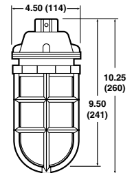
Pendant Incandescent
