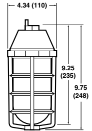
Pendant Incandescent
